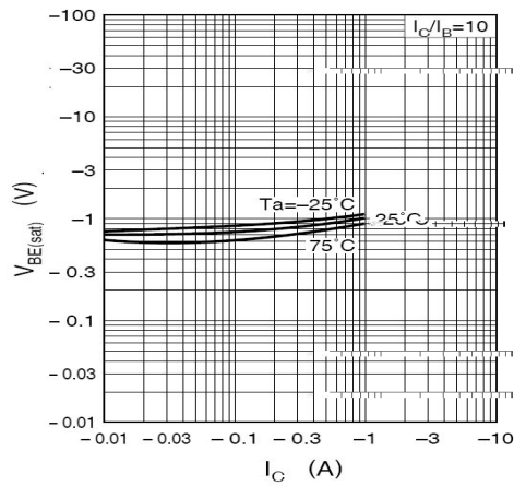
V_{BE(sat)} - I_C
