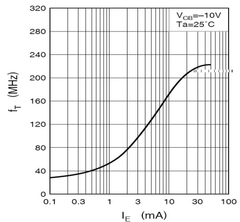
f_T - I_E
