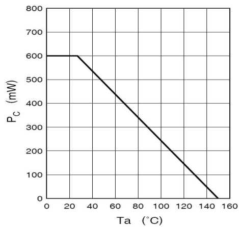
P_C - T_a
