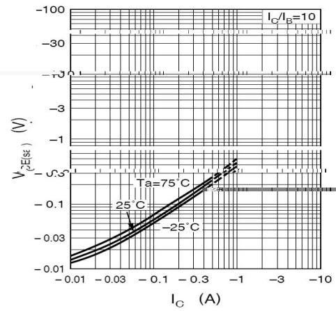
V_{CE(sat)} - I_C
