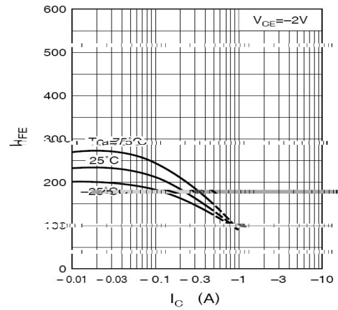
h_{FE} - I_C
