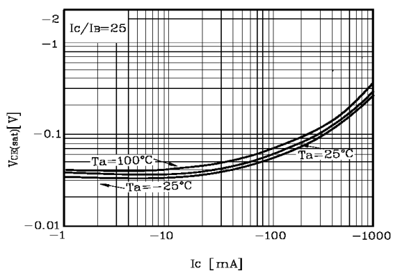
CE(SAT) - IC
