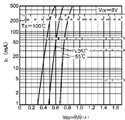
I_C - V_{BE}
