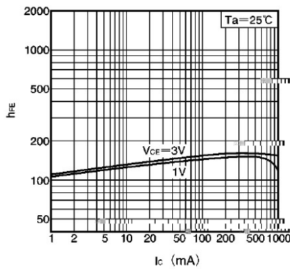
h_{FE} - I_C
