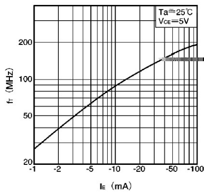
f_T - I_E
