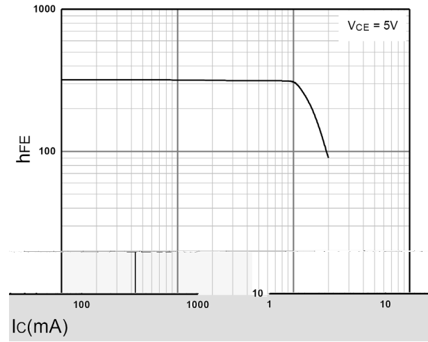
h_{FE} - I_C
